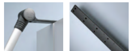
Die 12 (!) mm Ultraflach-Saugdüse arbeitet mit 8 Sauglöchern und deckt 22 x 4 cm Saugfläche in einem Zug ab.
